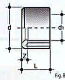
d Diámetro mayor d1 Diámetro menor L Longitud g Peso (gramos)
