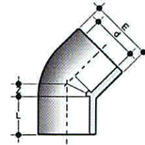
d Diámetro interno L Longitud campana E Diámetro externo g Peso (gramos)
