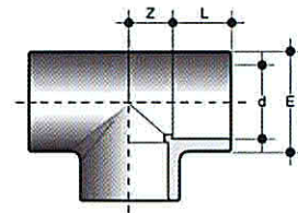
d Diámetro interno L Longitud campana E Diámetro externo g Peso (gramos)
