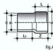
d Diámetro mayor d1 Diámetro menor L Longitud Campana L1 Longitud espiga E Diámetro exterior espiga
