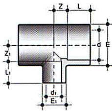
d Diámetro mayor d1 Diámetro menor L Longitud Campana L1 Longitud espiga E Diámetro externo
