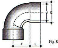
d Diámetro interno L Longitud campana E Diámetro externo g Peso (gramos)
