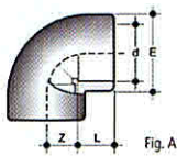
d Diámetro interno L Longitud campana E Diámetro externo g Peso (gramos)
