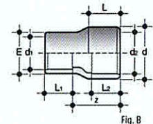
d Diámetro mayor d1 Diámetro menor L Longitud Campana L1 Longitud espiga E Diámetro exterior espiga
